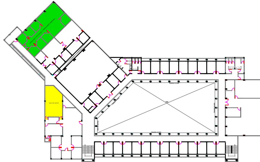
PLANTA ALTA
